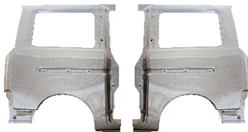
后叶子板 REAR FENDER-L/R L:Q22-5400030-DY R:Q22-5400040-DY
