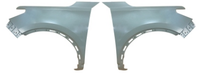
叶子板 FRONT FENDER-L/R L:553000205AADYJ R:553000206AADYJ
